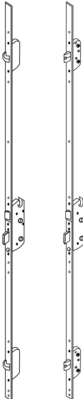
Hakenriegel des Standardsicherheitsstangengetriebes - für Drücker/Drückergarnituren
