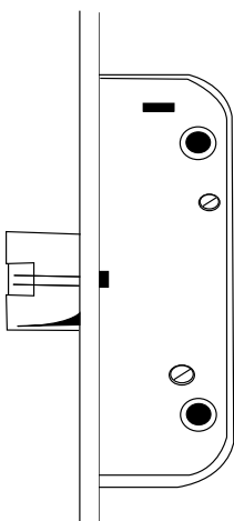
Automatisches Stangengetriebe - kann mit Knopf/Drückergarnitur verwendet werden
