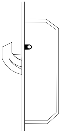
Hakenriegel des Standardsicherheitsstangengetriebes - für Drücker/Drückergarnituren
